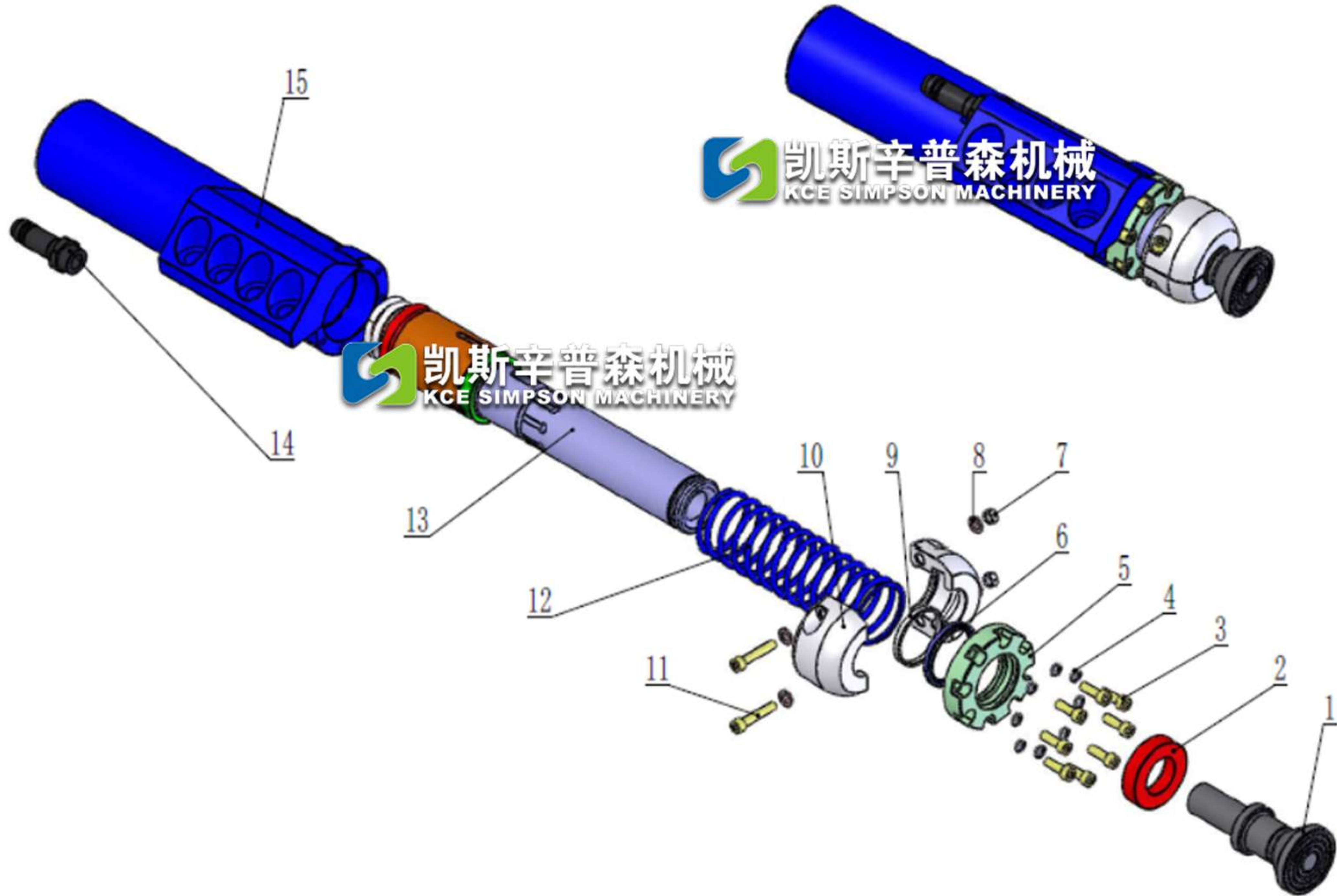
KCEN70plus高频气冲除芯锤爆炸图
